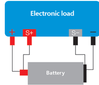
▲ Discharge Wiring
